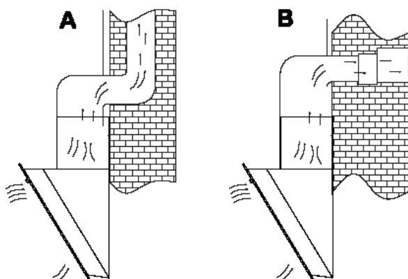
Fig. B Abluft ins Freie
