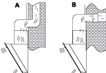
Fig. A Abluft über einen Luftschacht
